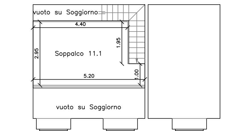
Planimetria soppalco appartamento 11 Sub_167 (scala 1:100 A3)
