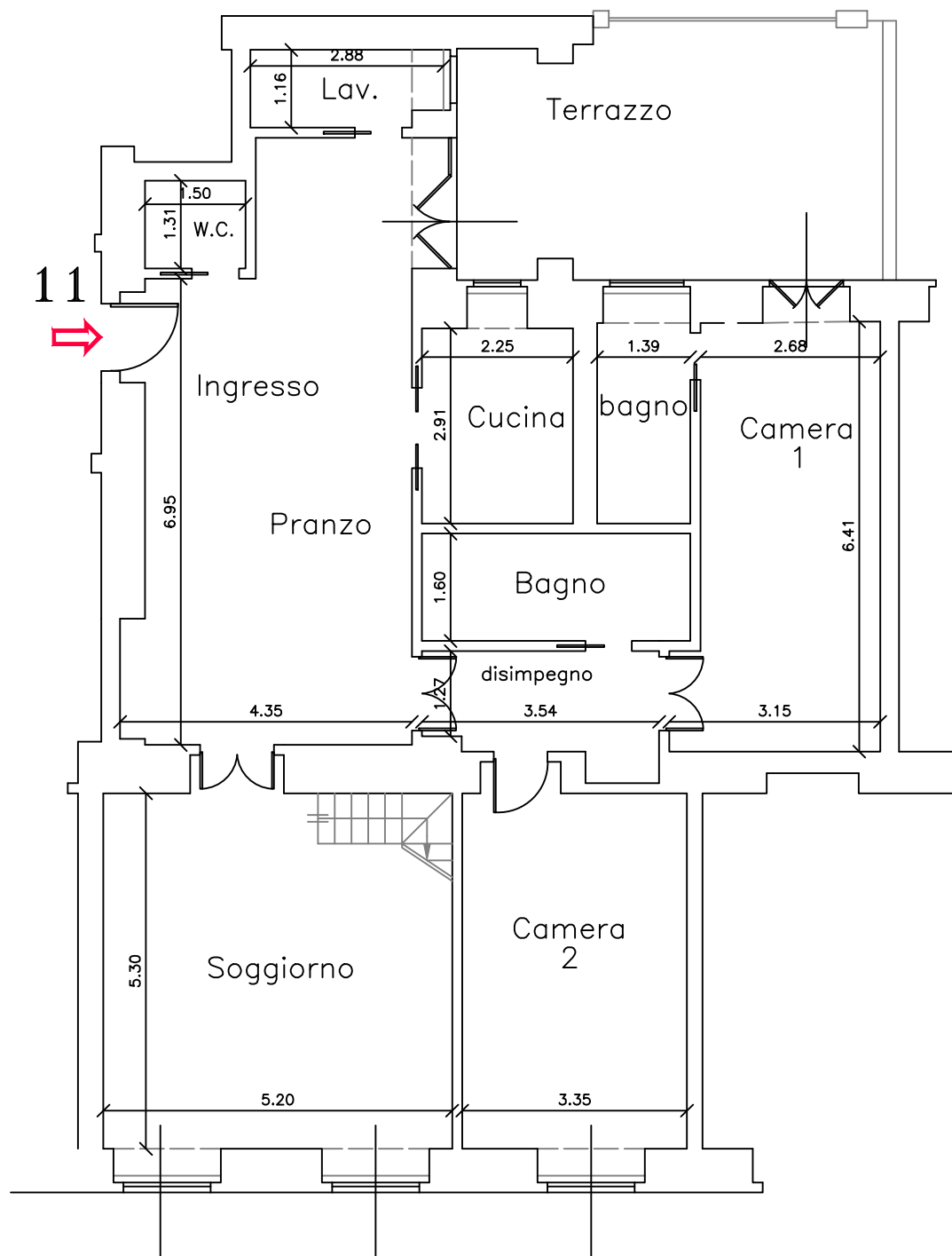
Planimetria appartamento 11 Sub_167 (scala 1:100 A3)
